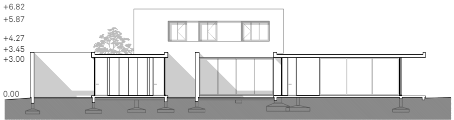
/Corte
