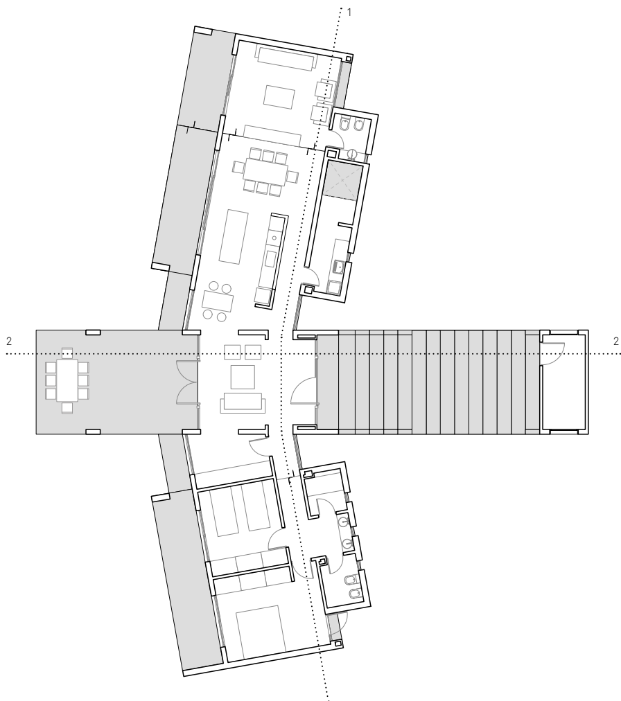
/Planta baja
