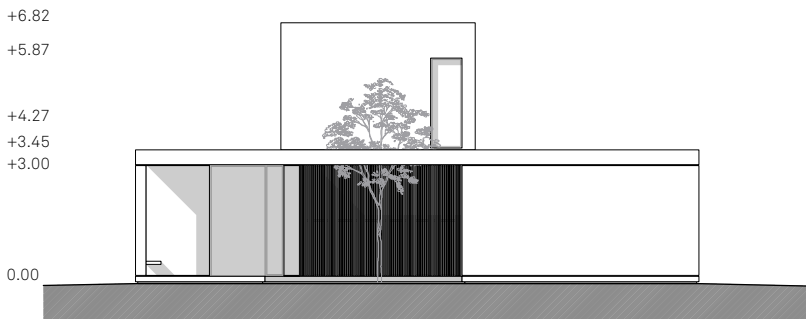
/Frente Sur
