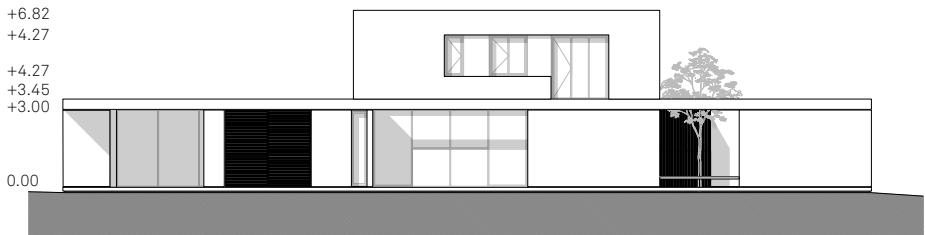
/Frente Oeste
